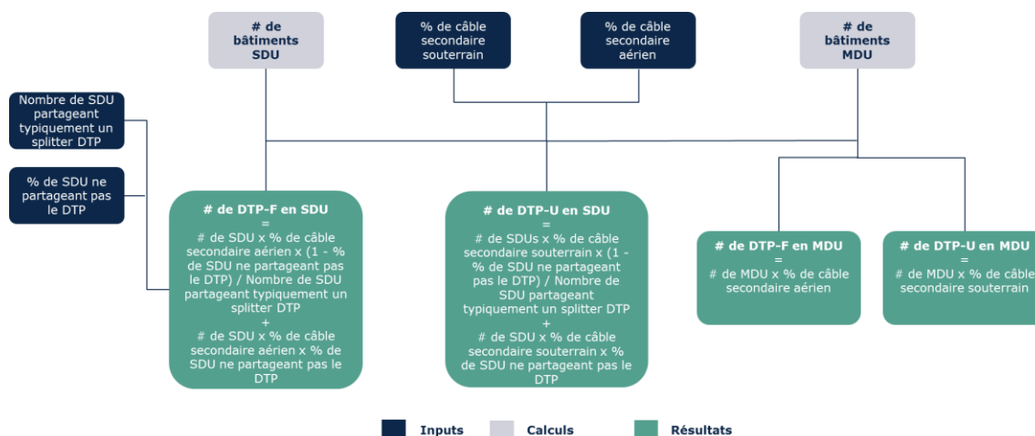
Figure 6.5 : Algorithme pour calculer le nombre de DTP selon la configuration [source : Axon Consulting]
