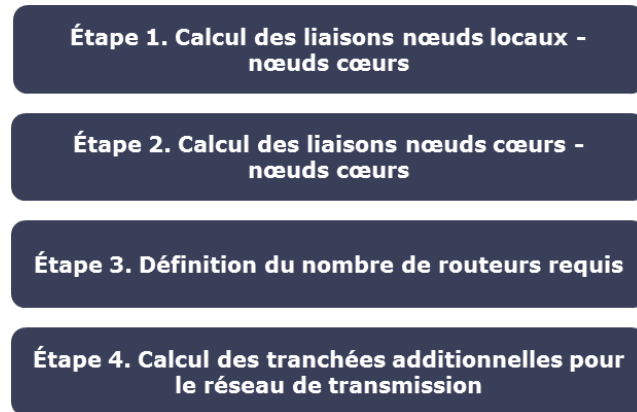
Figure 6.14 : Étapes pour le dimensionnement du réseau de transmission [source : Axon Consulting]
