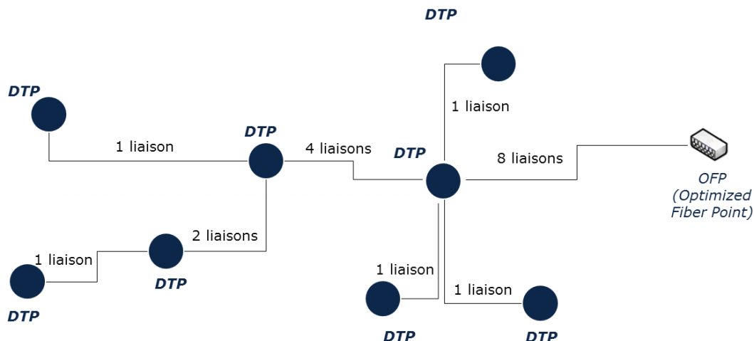
Figure 6.7 : Exemple d’agrégation de liaisons [source : Axon Consulting]
