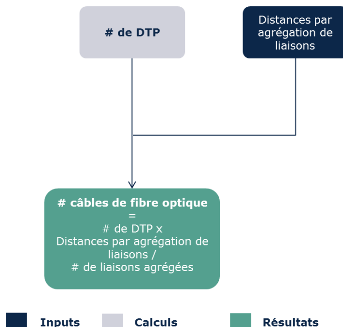
Figure 6.6 : Algorithme pour calculer le nombre de kilomètres de câble de fibre optique dans le réseau secondaire [source : Axon Consulting]
