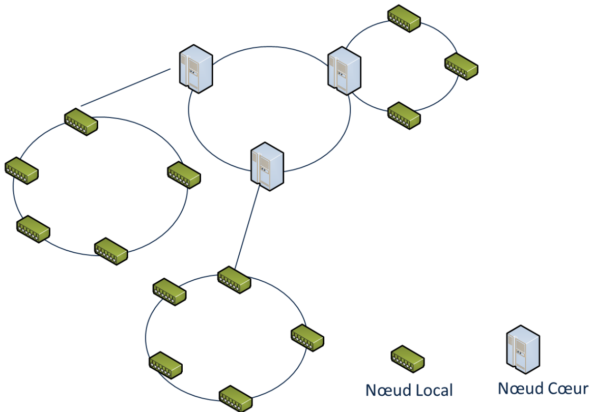
Figure 6.13 : Aperçu de l'architecture générale prise en compte dans le réseau de transmission [source : Axon Consulting]
