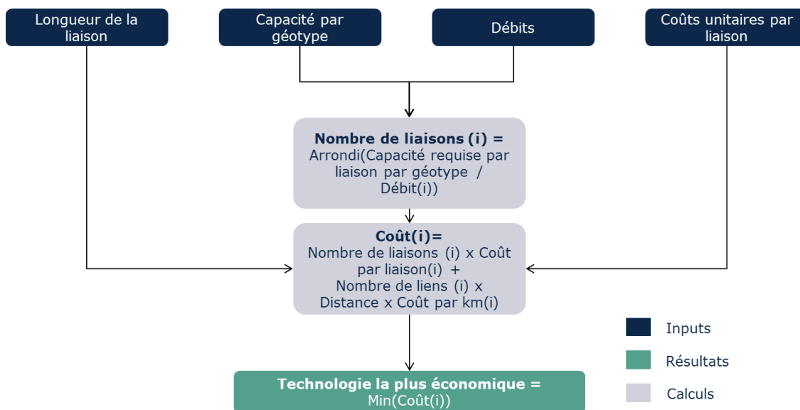
Figure 6.15 : Calcul de la configuration optimale de liaisons. [source : Axon Consulting]
