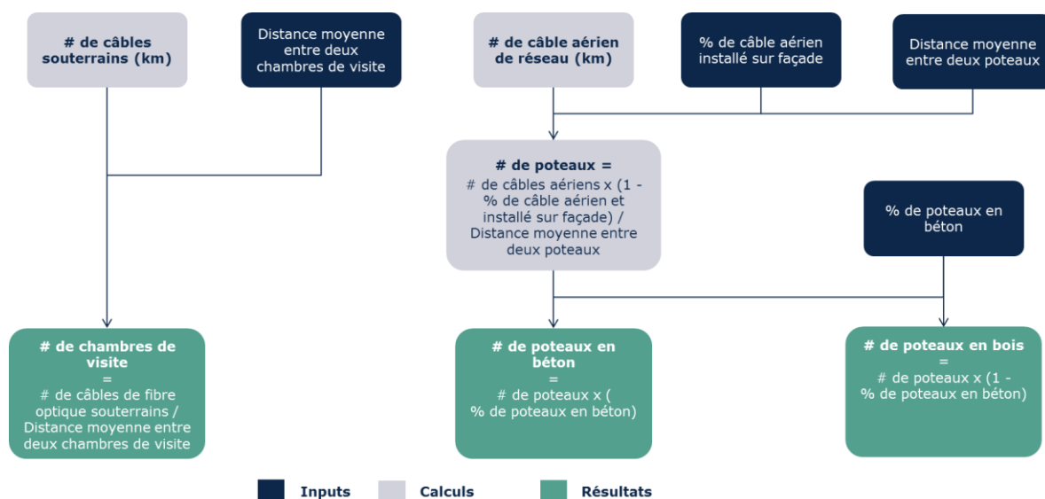
Figure 6.10 : Algorithme pour calculer le nombre de chambres de visite et de poteaux dans le réseau secondaire [source : Axon Consulting]
