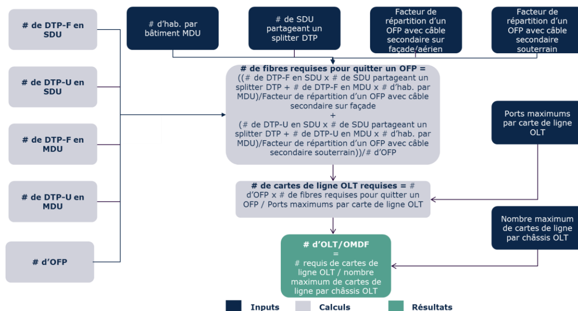
Figure 6.12 : Algorithme pour calculer le nombre d'OLT et d'OMDF [source : Axon Consulting]
