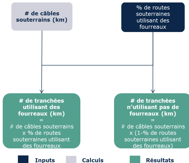
Figure 6.9 : Algorithme pour le calcul des kilomètres de tranchées utilisant ou non des fourreaux au sein du réseau d'accès [source : Axon Consulting]
