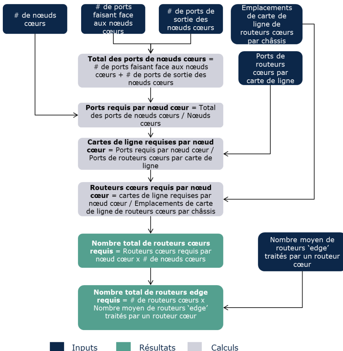
Figure 6.17 : Algorithme utilisé pour calculer le nombre de routeurs cœurs nécessaires [source : Axon Consulting]
