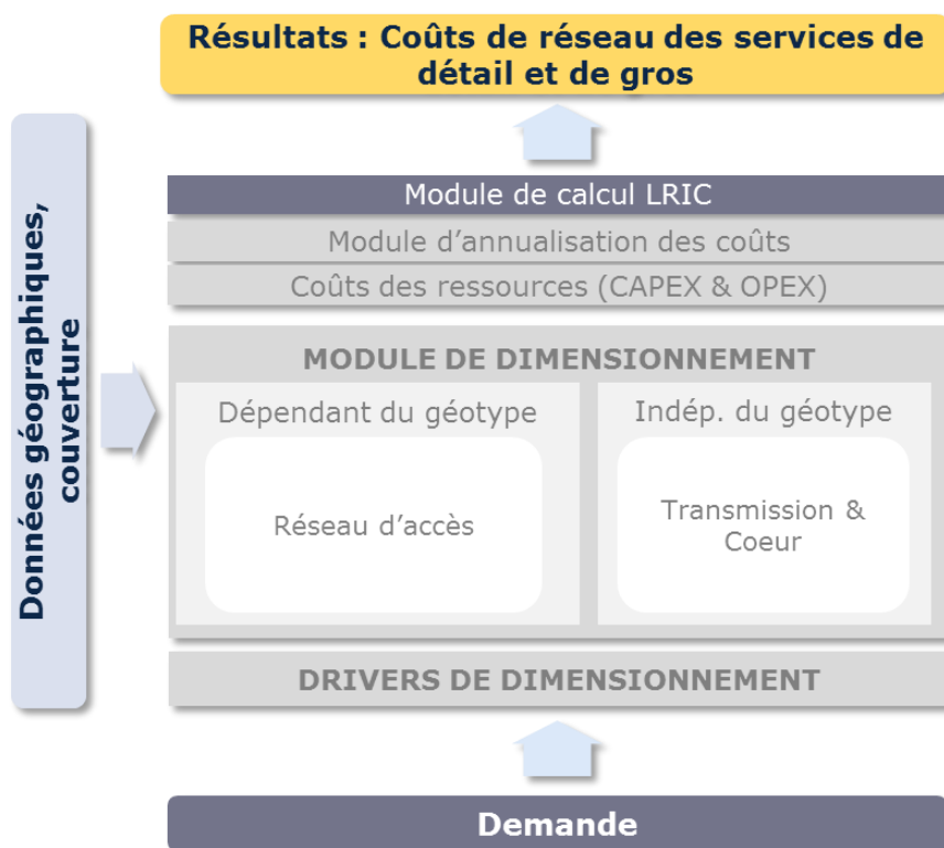
Figure 2.1 : Structure du modèle [source : Axon Consulting]
