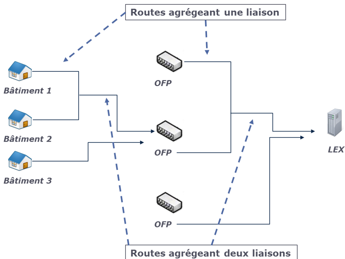
Figure 5.5 : Exemple de connexion d'éléments de réseau utilisant une topologie arborescente de distance minimum [source : Axon Consulting]
