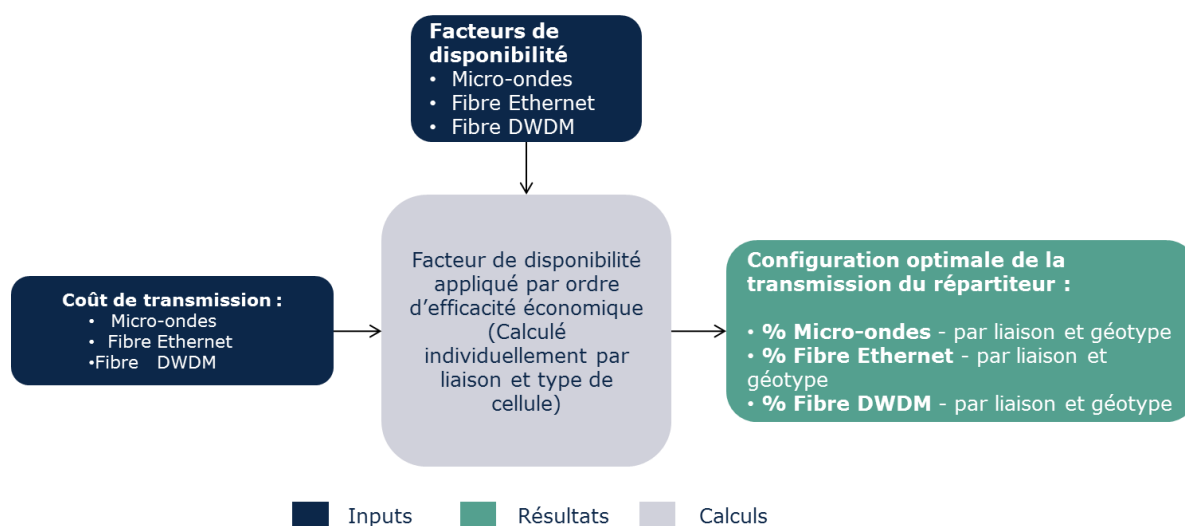
Figure 6.16 : Définition du réseau de transmission optimal [source : Axon Consulting]
