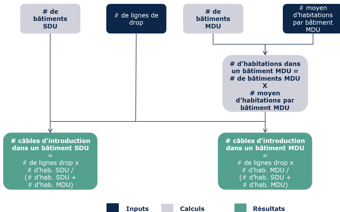
Figure 6.4 : Algorithme pour le calcul du nombre d'unités d'introduction dans les SDU et MDU [source : Axon Consulting]
