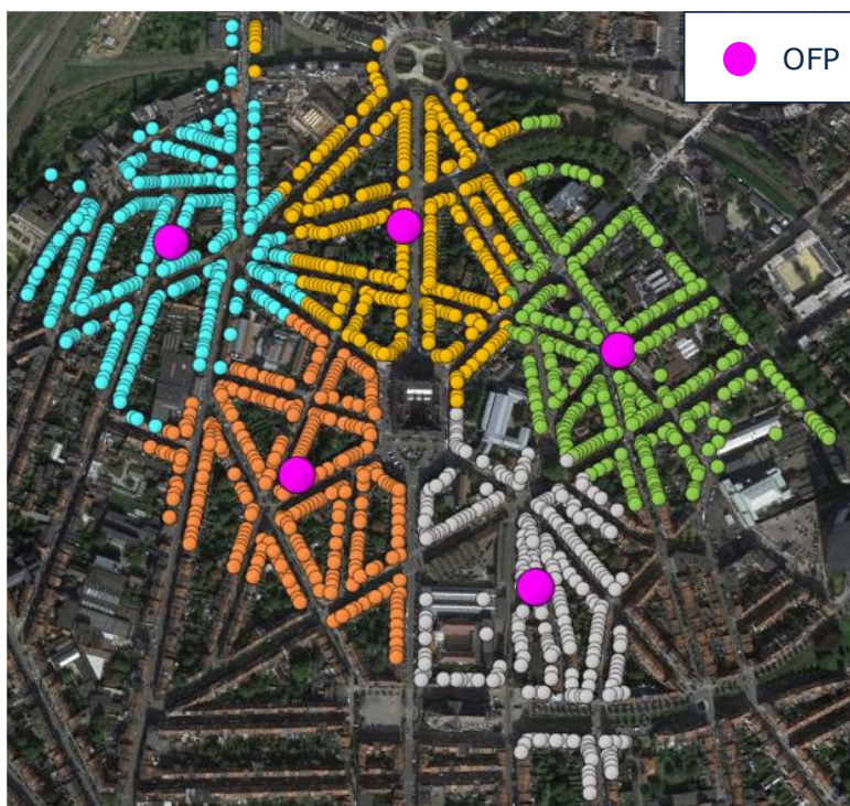
Figure 5.3 : OFP qui devraient être déployés pour une zone située dans un géotype URBAIN [source : Axon Consulting]
