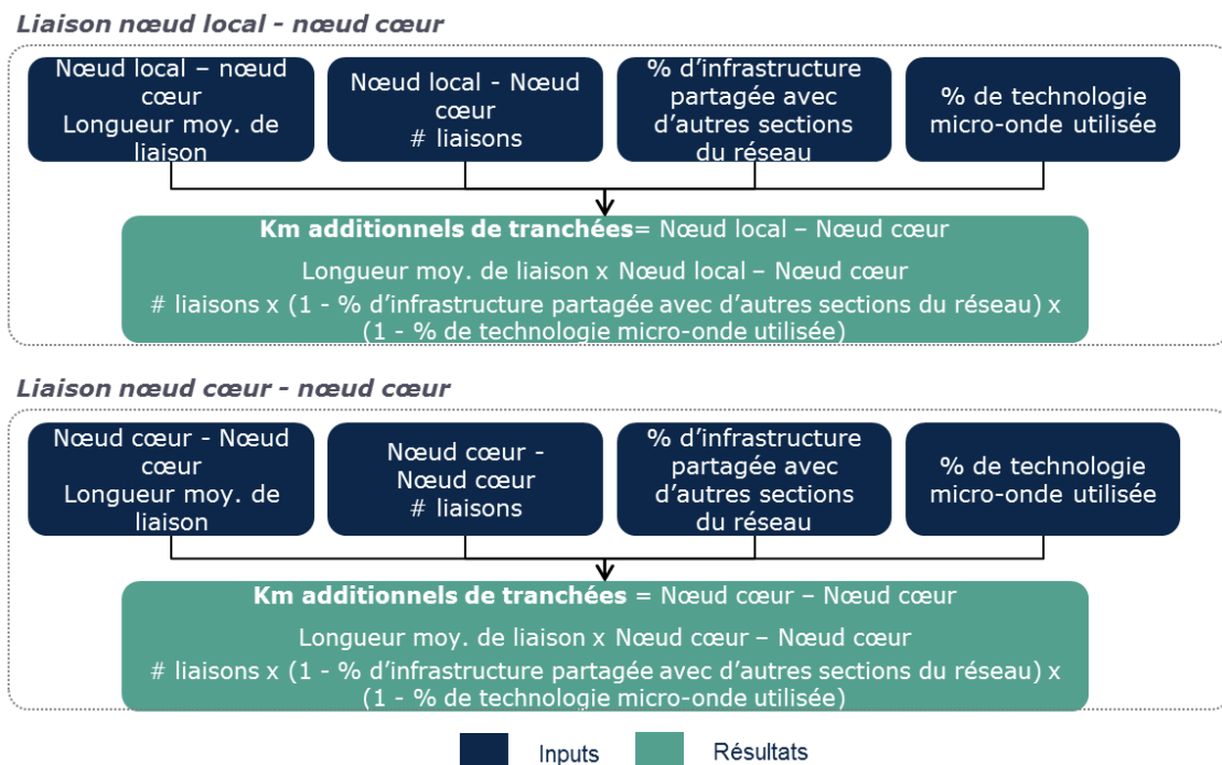
Figure 6.18 Calcul des tranchées additionnelles à déployer par type de liaison [source Axon Consulting]
