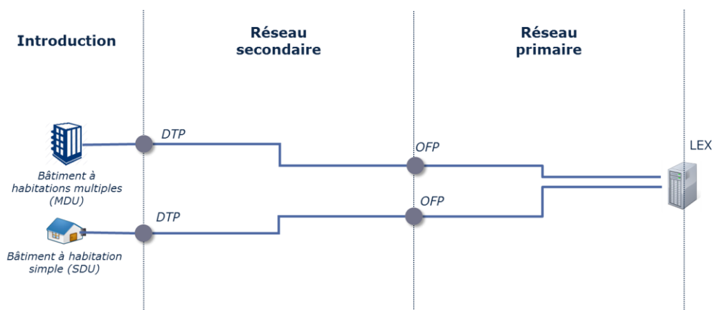
Figure 6.1 : Architecture du réseau d'accès modélisé [source : Axon Consulting]
